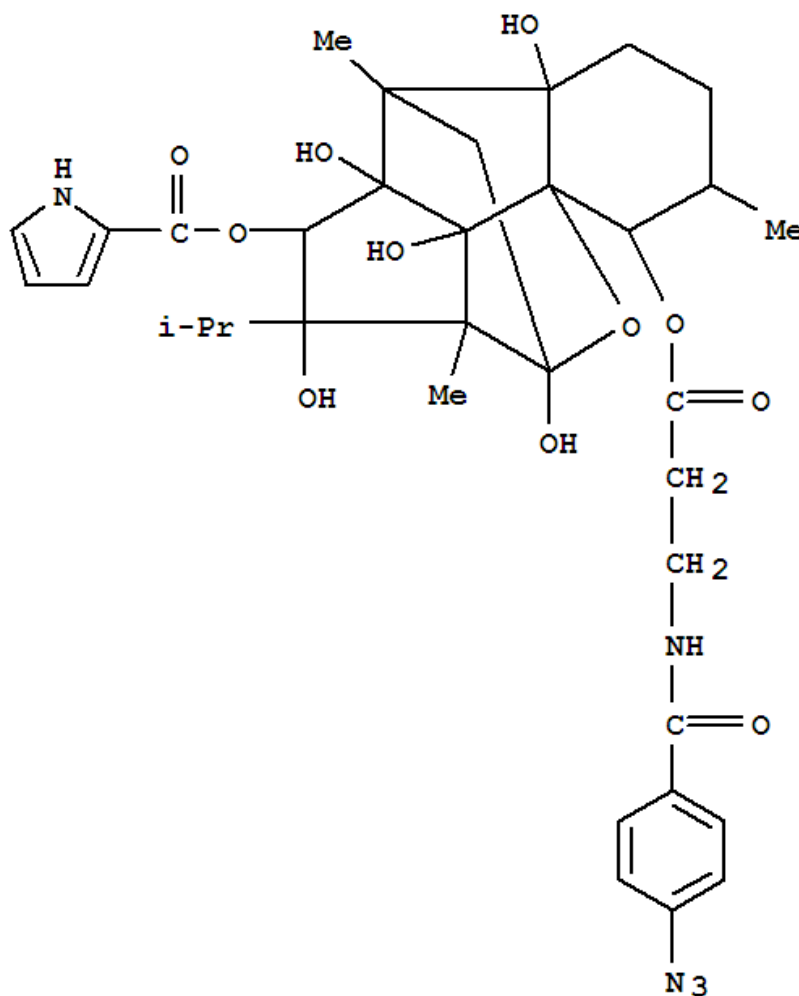
分子结构:
